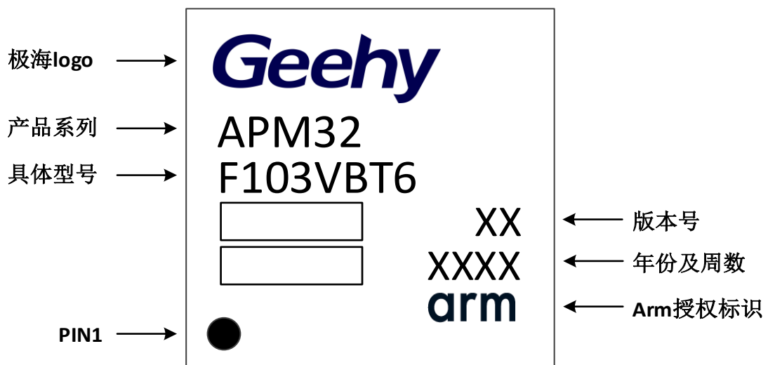
图23 LQFP100 - 100 引脚，14 x 14mm 封装标识
