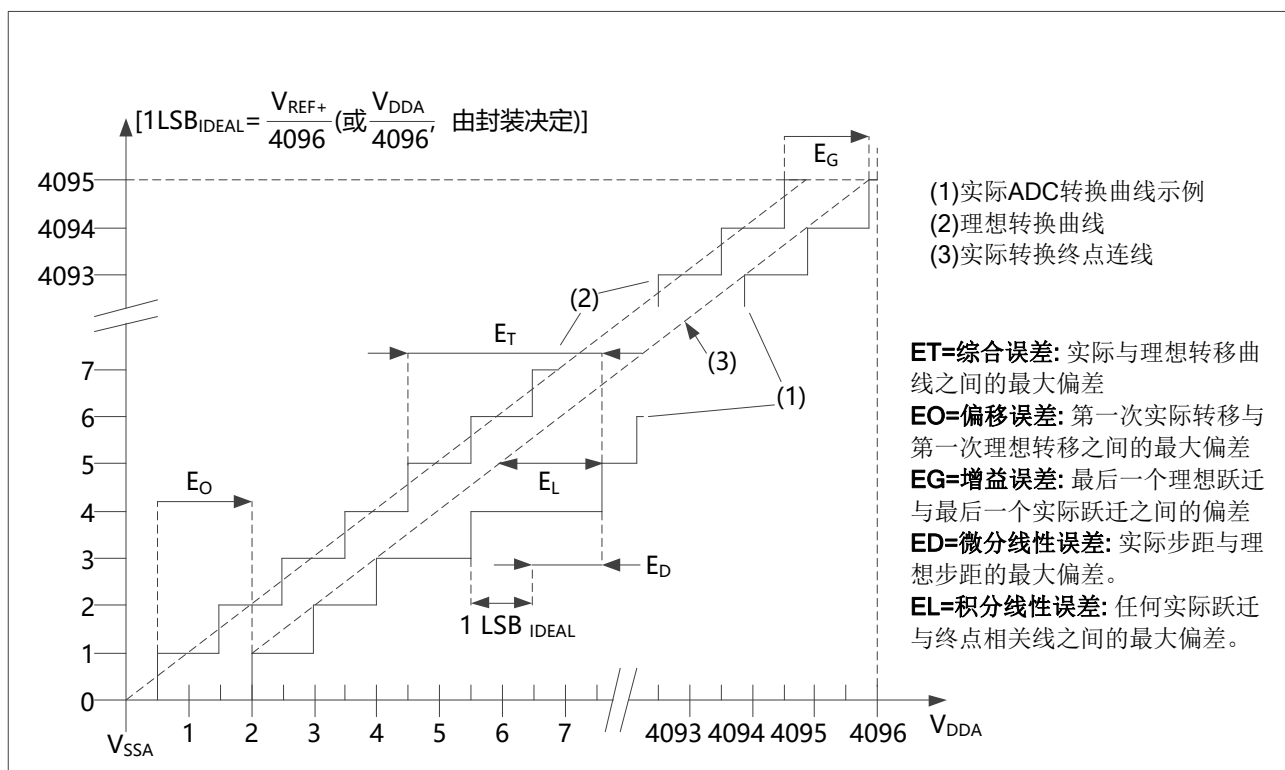
图20 ADC 精度特性
